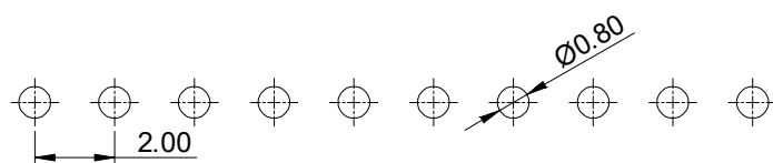
P.C.B Hole Layout
