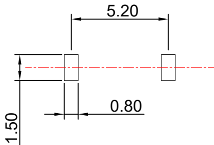
适用线路板(PCB LAYOUT)
