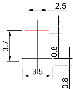
PCB 开孔尺寸
